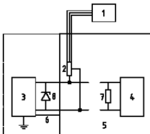
1-示波器或等效设备 2-电压探头 3-电源内阻为 R_i 的试验脉冲发生器 4-DUT 5-接地平板 6-接电线（试验脉冲3的最大长度为100mm） 7-任意电阻 8-任意二极管桥
