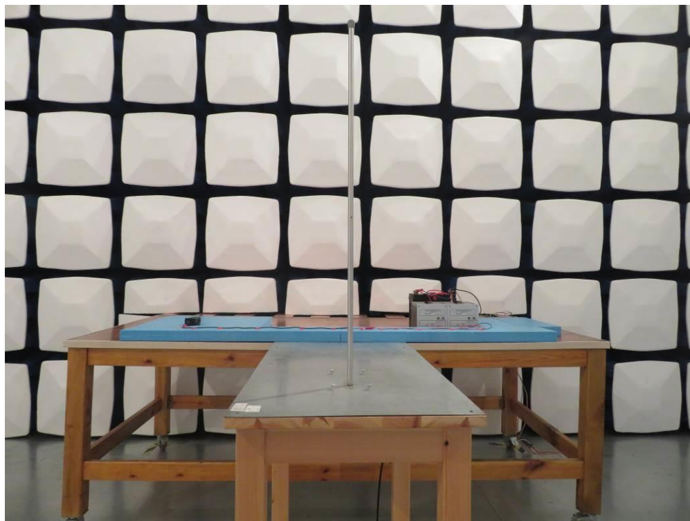
杆天线测试
