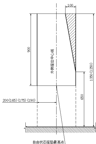
图8 座椅上方的自由空间
