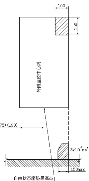
图9 外侧座椅空间的允许侵入
